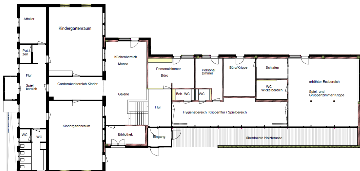
GRUNDRISS EG M 1:125
