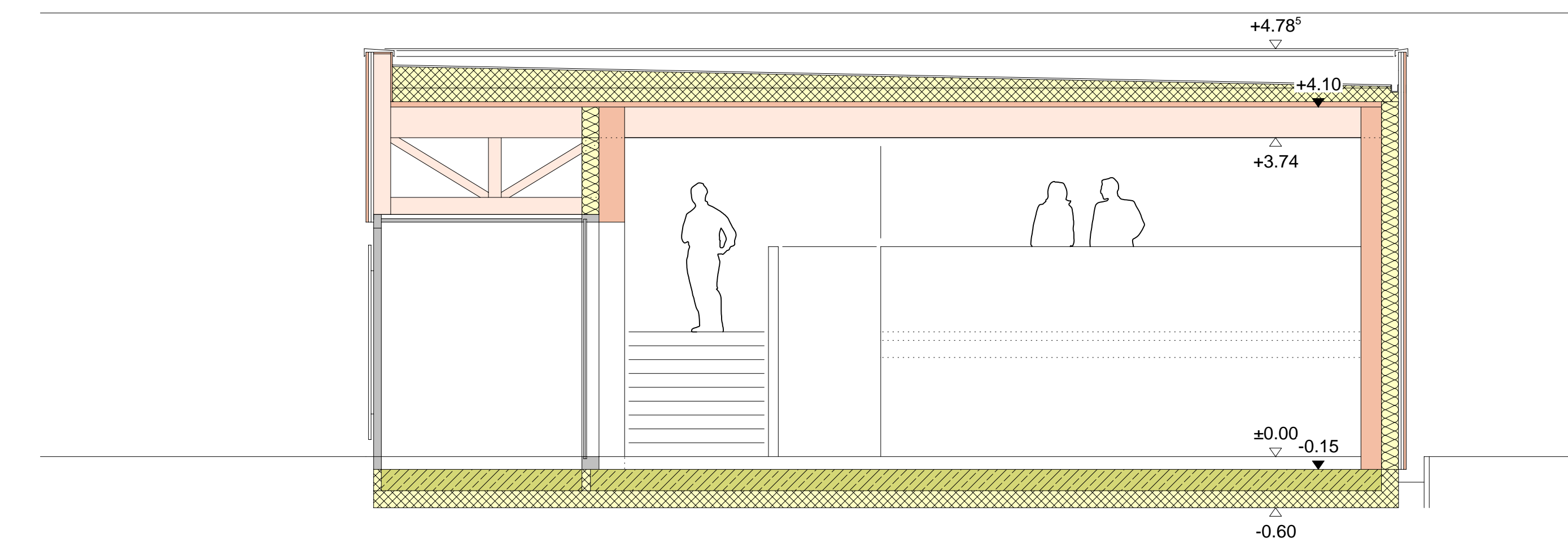
QUERSCHNITT A // 1_50
